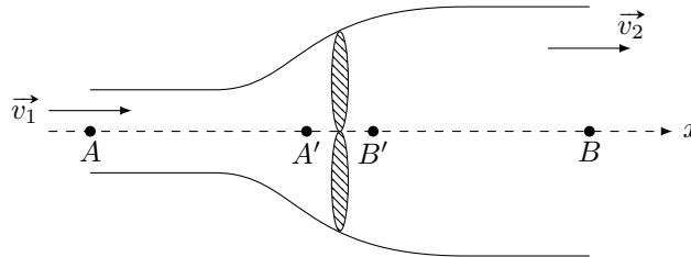
Tube de courant en présence de l'éolienne
